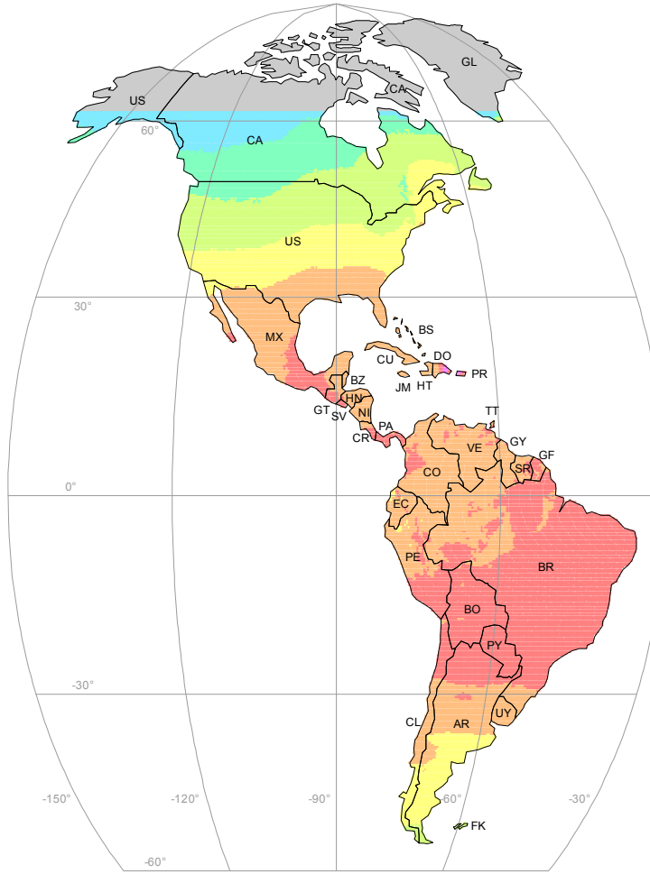
Mollweide-Projektion Zentralmeridian 90° West
